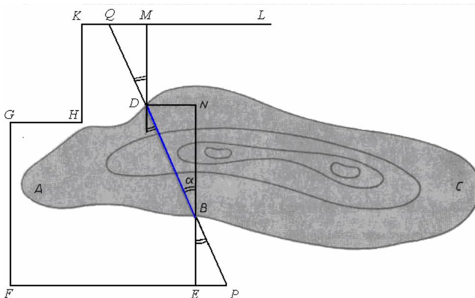
Рис. 30. Геометрические построения на плане местности при прокладке Самосского тоннеля.
