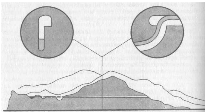
Рис. 29. Самосский тоннель. Поперечное сечение горы Кастро (внизу), поперечное сечение тоннеля и водостока (слева) и горизонтальный план тоннеля в месте стыковки (справа).
