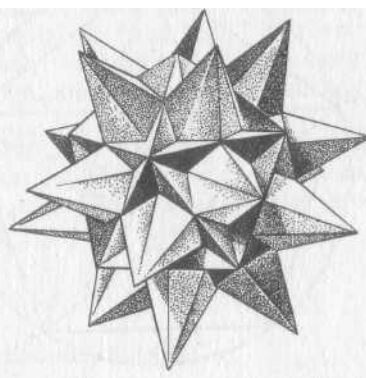
Рис. 49. Седьмая звездчатая форма тела Архимеда — икосододекаэдр.
