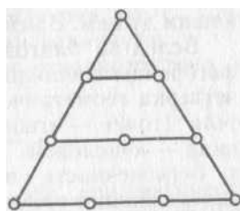
треугольное число 10
