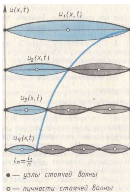
Рис. 77. Четыре первые стоячие волны (гармоники) колеблющейся струны.
