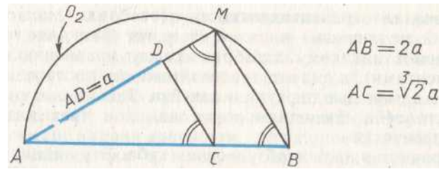
Рис. 70. Треугольник Архита.
