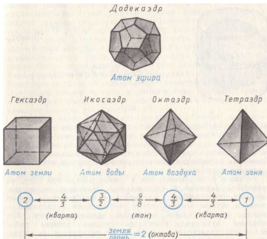
Рис. 81. Правильные многогранники и их физическая и музыкальная интерпретация по Платону.
