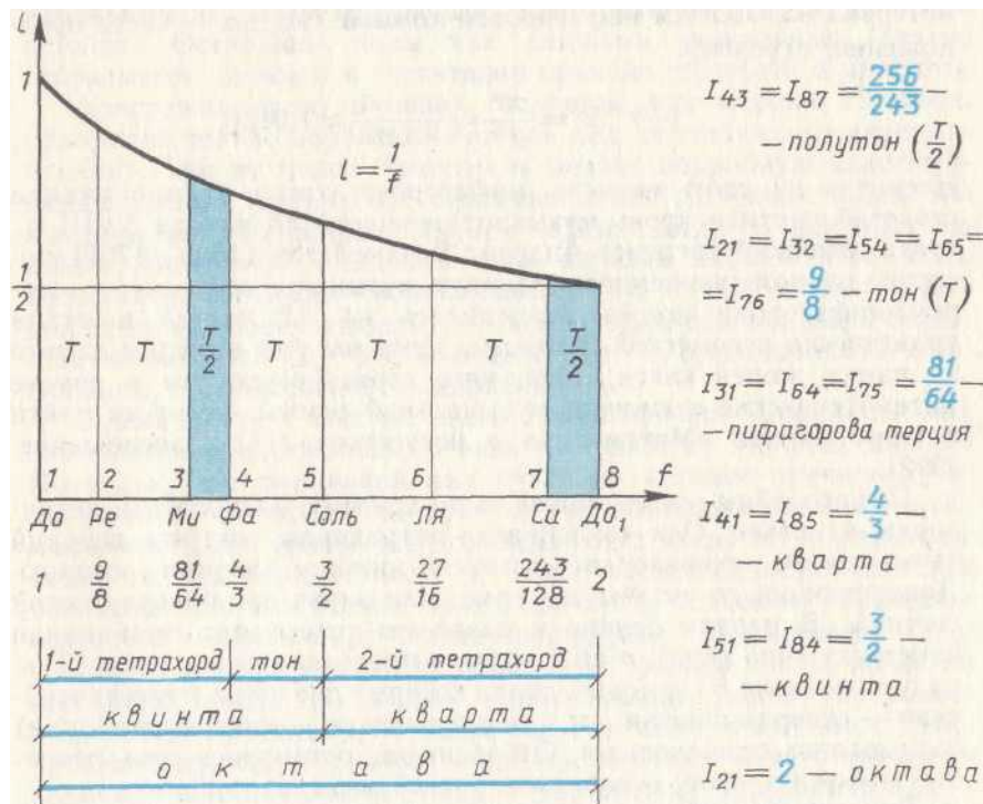
Рис. 76. Пифагоров строй лидийской гаммы и его математические характеристики.
