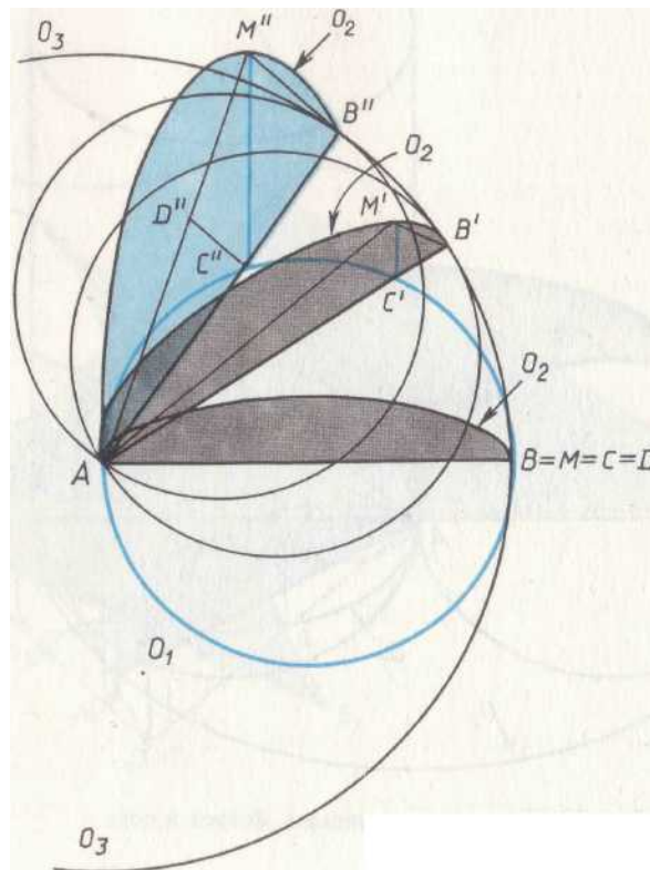
Рис. 71. Пересечение цилиндра и тора.
