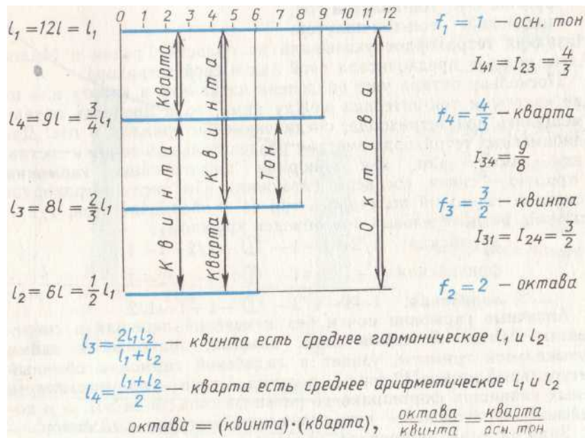
Рис. 75. Деление струны монохорда ( l_1 ) на части, образующие с ней совершенные консонансы: октаву ( l_2 ), квинту ( l_3 ) и кварту ( l_4 ) и соотношения между ними.
